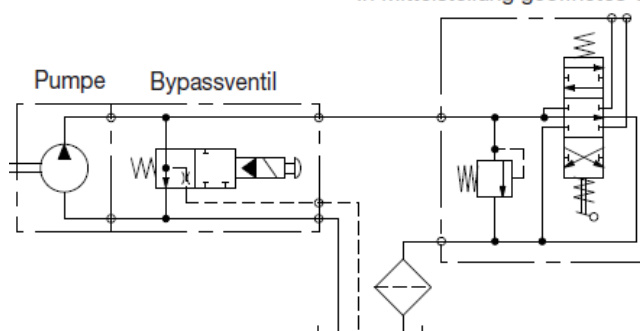
In Mittelstellung geöffnetes Ventil
